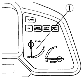
(1) Fuel meter
