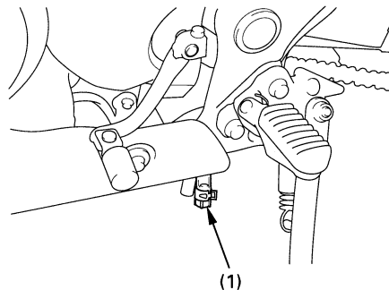
(1) Kurbelgehäuse-Entlüftungsschlauchstopfen
