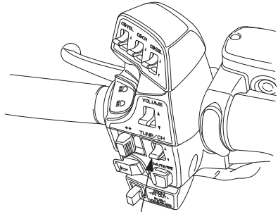
TUNE/CH lever
