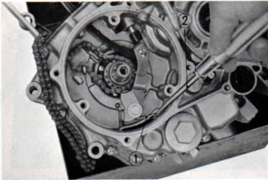
Fig. 79 Pose du tendeur de chaîne ① Ressort ② Tournevis
