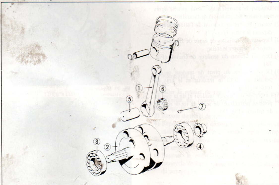
Fig. 81 ① Bielle ② Vilebrequin ③ Roulement 6305 ④ Pignon de distribution ⑤ Maneton ⑥ Cage ⑦ Clavette
