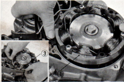
Fig. 80 Pose de l'alternateur ① Stator ② Caoutchouc de faisceau ③ Joint torique
