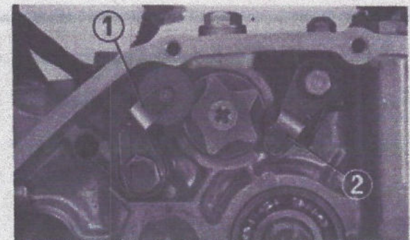
Fig. 3-61 (1) Bras de butée de tambour sélecteur (2) Bras de butée de point mort
