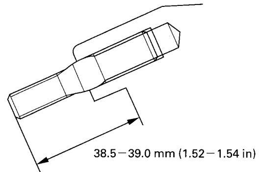
Exhaust pipe stud bolt:
