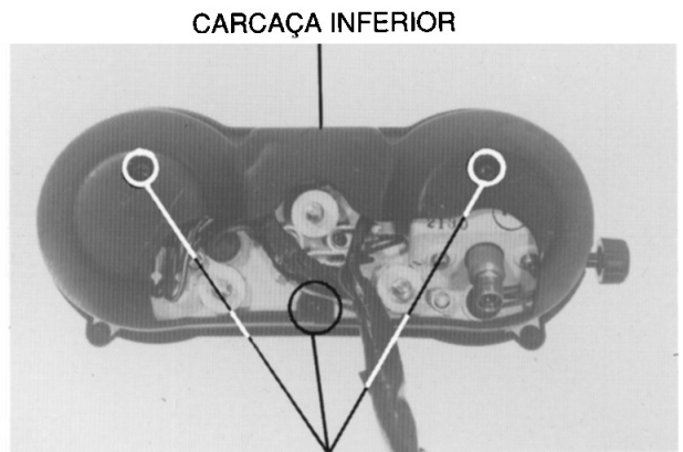
PARAFUSOS
